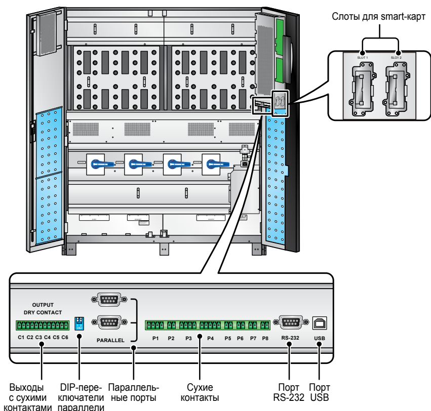
Рис. 4-1. Коммуникационные интерфейсы
