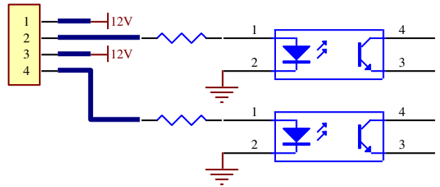
Рис.3-12 Входные контакты
