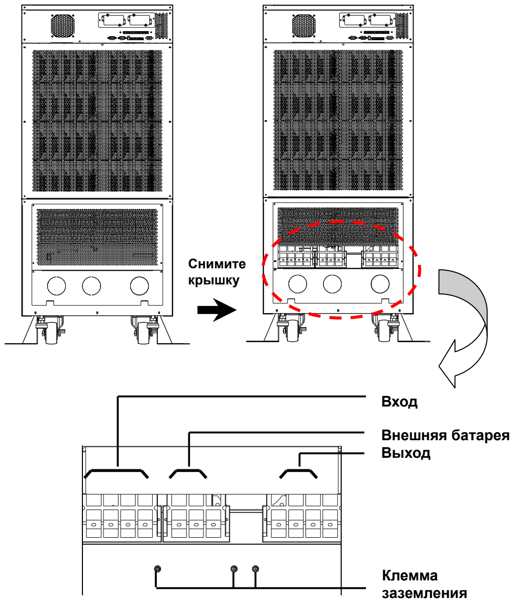
Рис.4-3 Клеммная коробка
