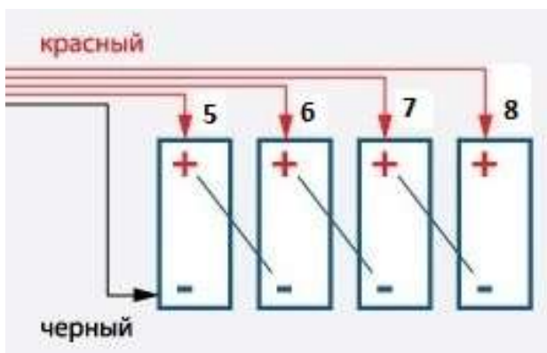
Аккумуляторы 2 В №№ 2÷8
