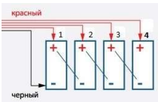
Аккумуляторы 2 В №№ 1÷4
