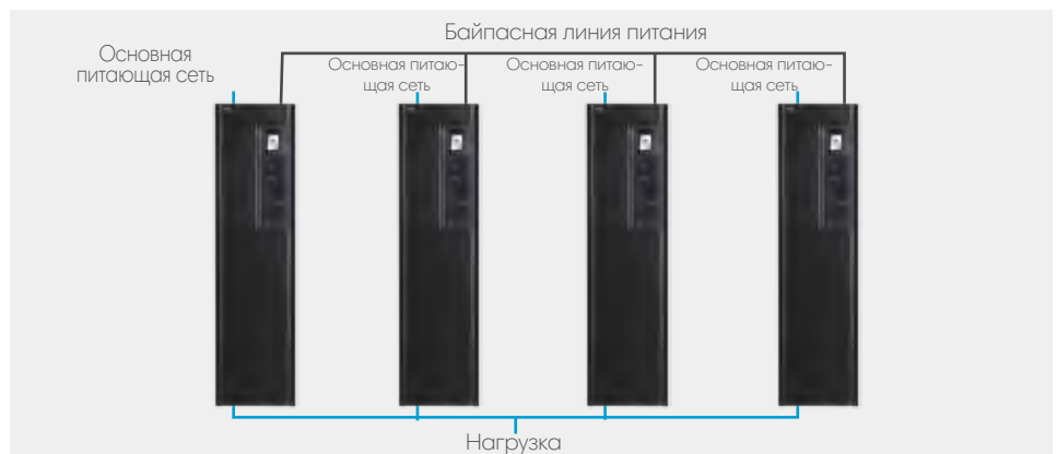
Liebert EXS, параллельная конфигурация
