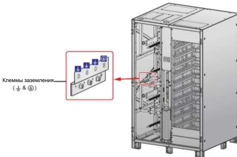
Рисунок 2-9: Клеммы заземления
