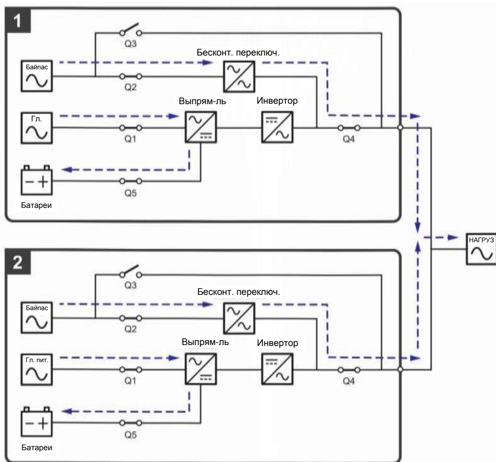
Рисунок 3-24: Схема байпасного режима, подключение параллельных ИБП к двум линиям питания
