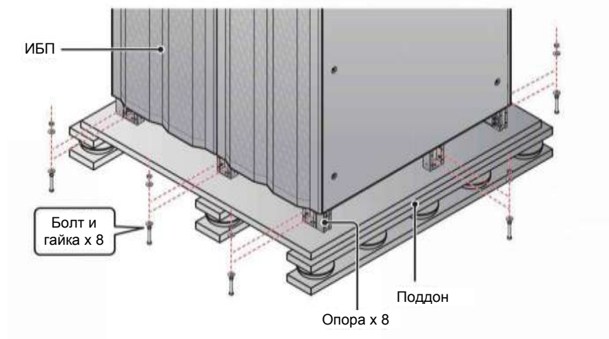
Рисунок 5-2: Расположение опор, болтов и гаек
