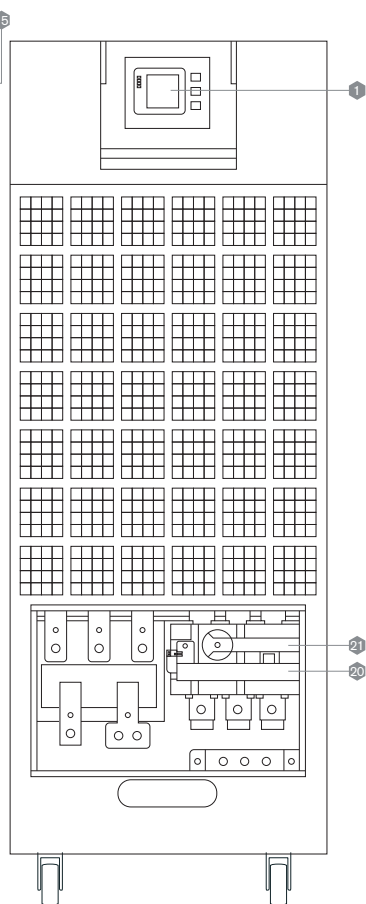
Вид спереди: YDC33200H (200 кВА)
