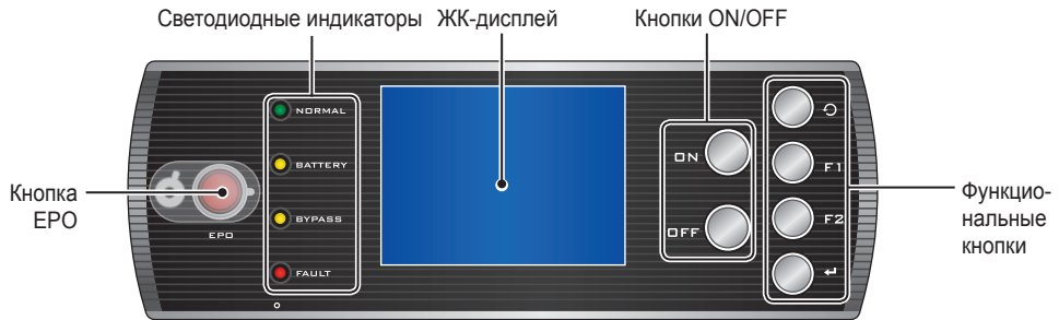
Рис. 2-8. Панель управления
