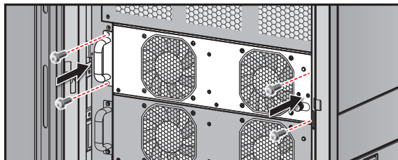
Рис. 7-5. Фиксация винтами
