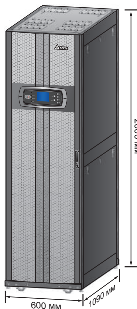
Рис. 2-2. Размеры
