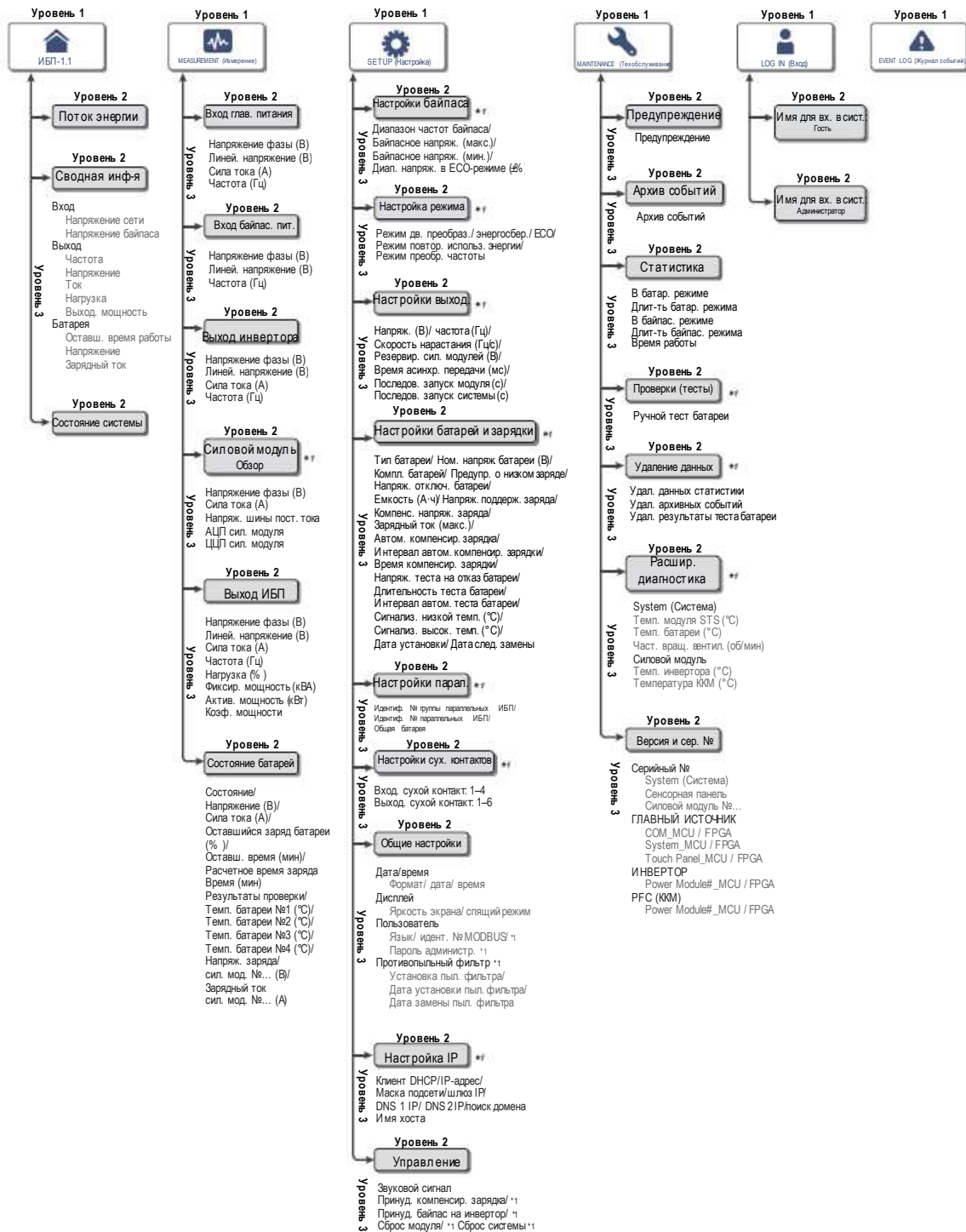
Рисунок 7-1: Иерархия ЖК-дисплея
