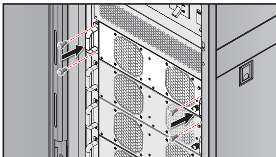
Рис. 5-20: Фиксация винтами
