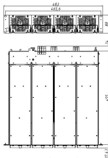
Модульный каркас PS2000K
