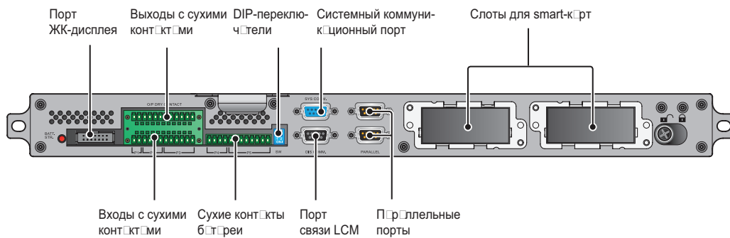
Рис. 4-2. Коммуникационные интерфейсы
