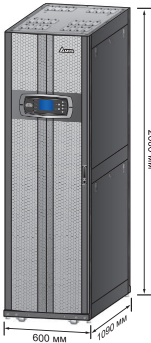
Рис. 2-2. Размеры
