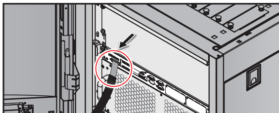
Рис. 5-33. Отсоединение кабеля ЖК-дисплея
