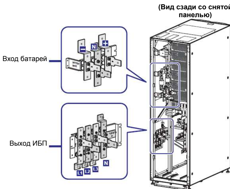
Рисунок 5-12: Клеммы: вход для подключения батарей и выход ИБП
