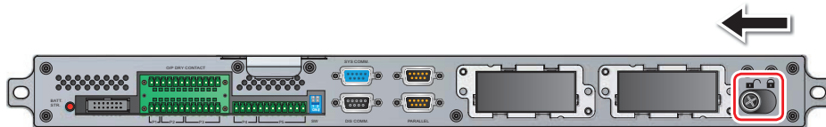
Рис. 5-31. Разблокировка защёлки
