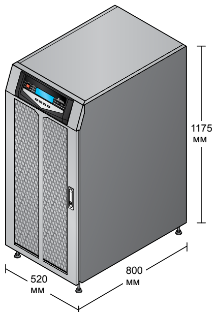
Рис. 3-1. Внешний вид и размеры ИБП 60/80 кВА
