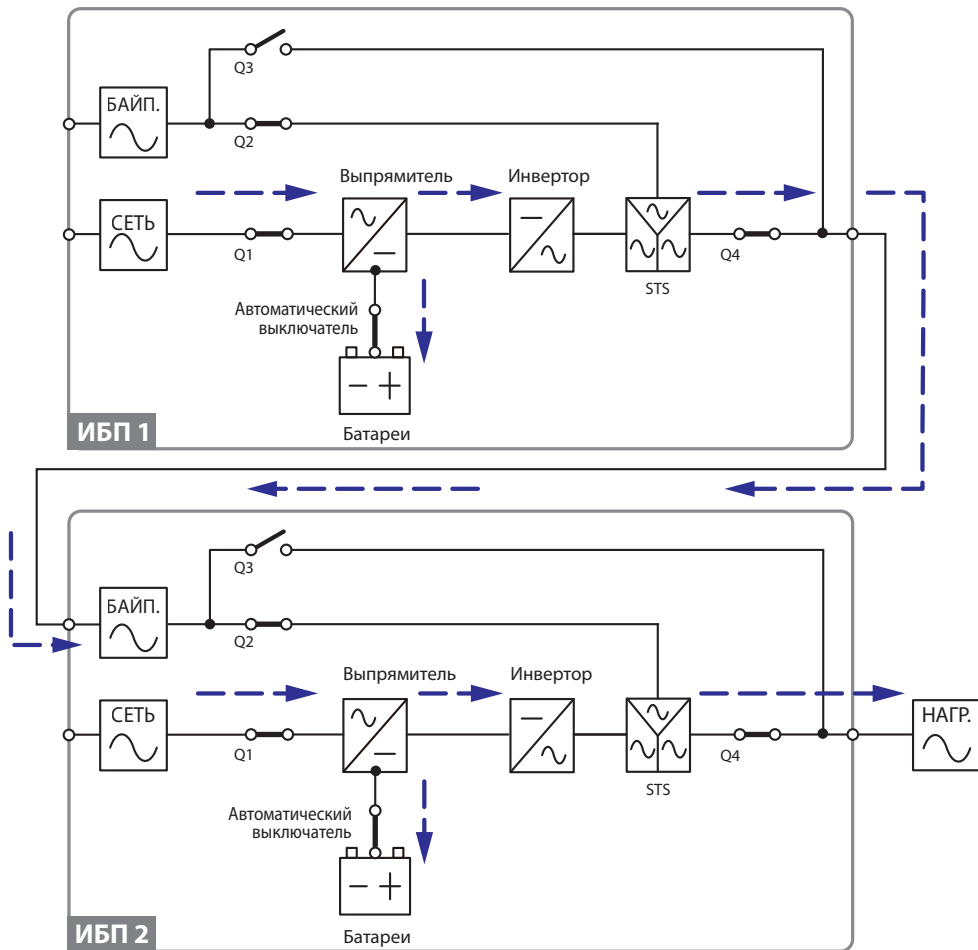
Рис. 3-10. Последовательное резервирование
