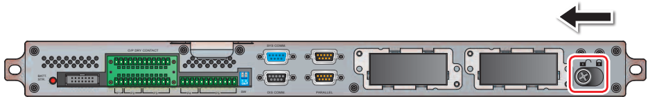
Рис. 7-15. Разблокировка защёлки
