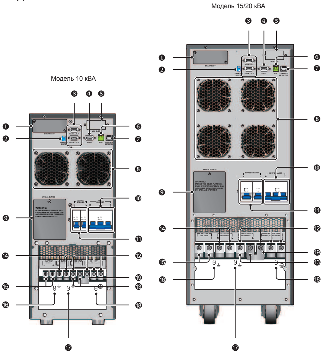
Рис. 3-3. Задняя панель
