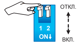
Рис. 5-2. DIP-переключатели параллели
