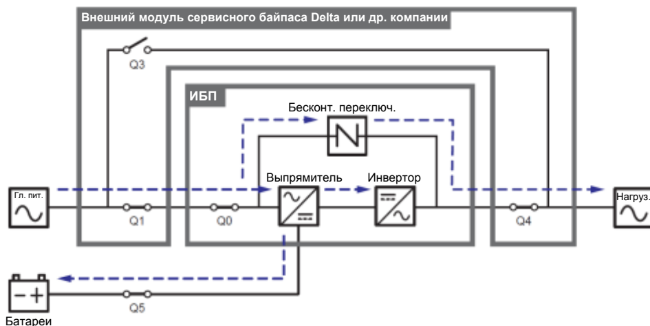
Рисунок 3-7: Схема ESO-режима, подключение одного ИБП к одной линии
