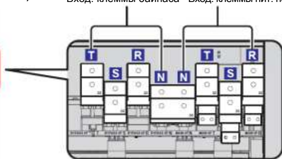
Рисунок 5-6: Расположение задней панели и винтов
