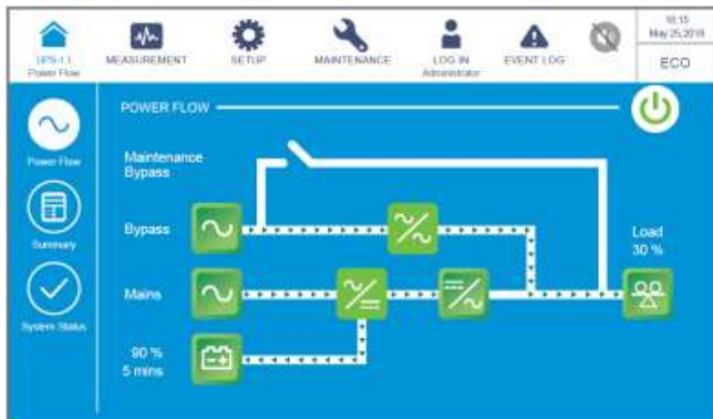
Рисунок 6-26: Экран ECO-режима
