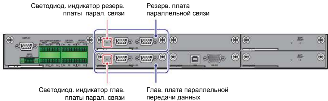
Рисунок 4-11: Расположение главной и резервной плат параллельной передачи данных и их светодиодных индикаторов
