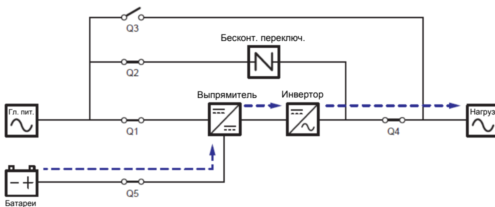
Рисунок 3-2: Схема батарейного режима, подключение одного ИБП к одной линии питания
