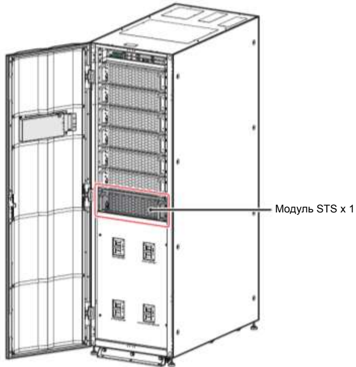
Рисунок 5-32: Расположение STS-модуля
