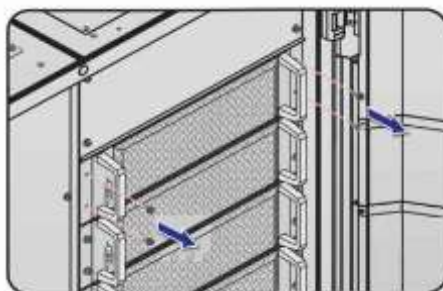
Рисунок 5-39: Снятие 4 винтов
