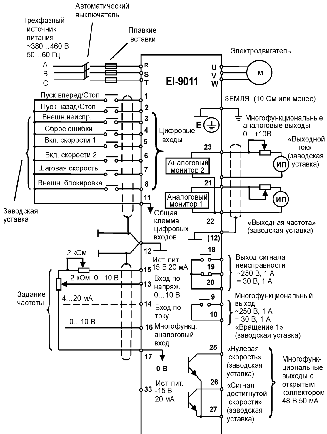
Рис. 4. Схема подсоединения
