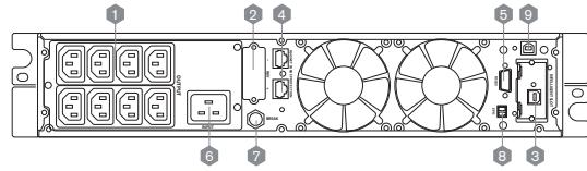
Вид сзади: UDC9102 (2 кВА)
