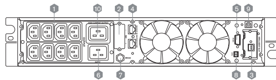
Вид сзади: UDC9103 (3 кВА)
