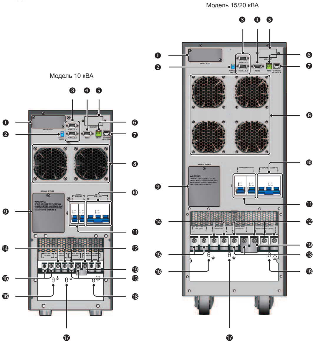
Рис. 3-3. Задняя панель
