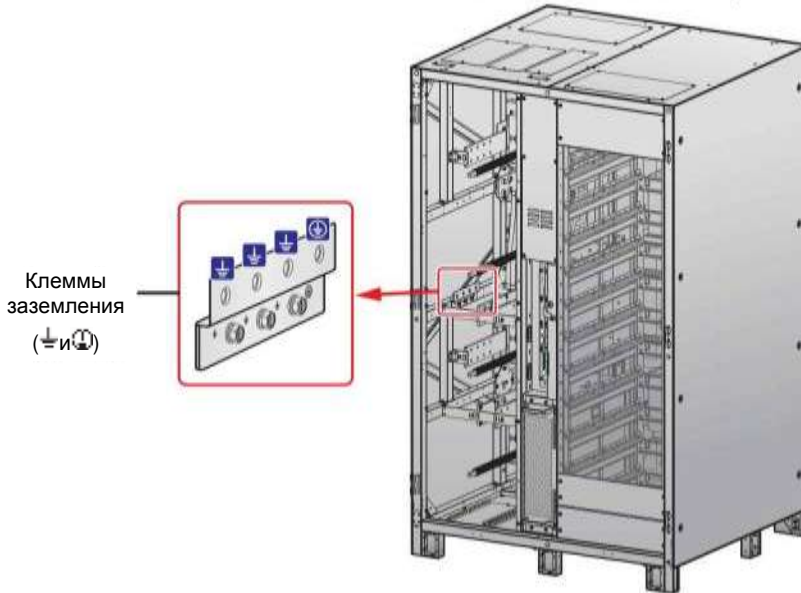
Рисунок 5-10: Клеммы заземления
