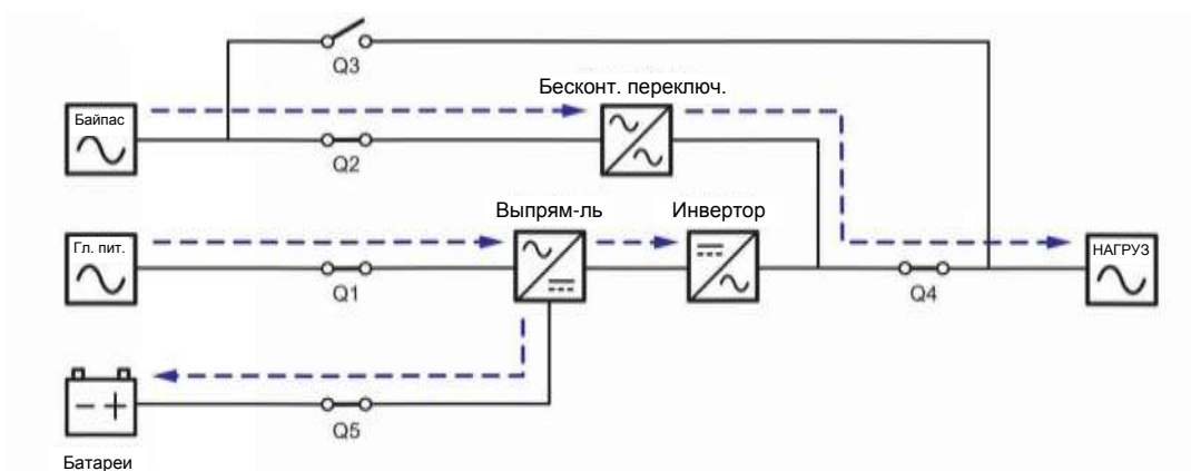
Рисунок 3-19: Схема ESO-режима, подключение одного ИБП к двум линиям питания
