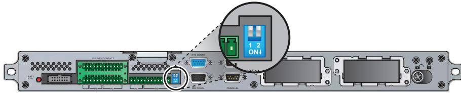
Рис. 6-2. DIP-переключатели
