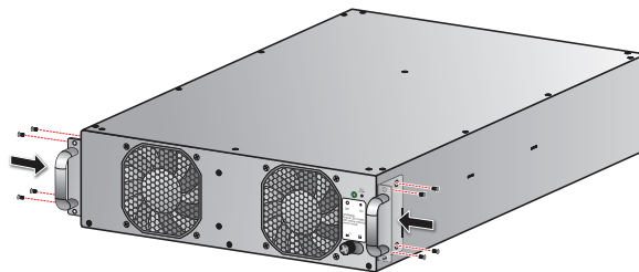
Рис. 5-18: Крепление ручек
