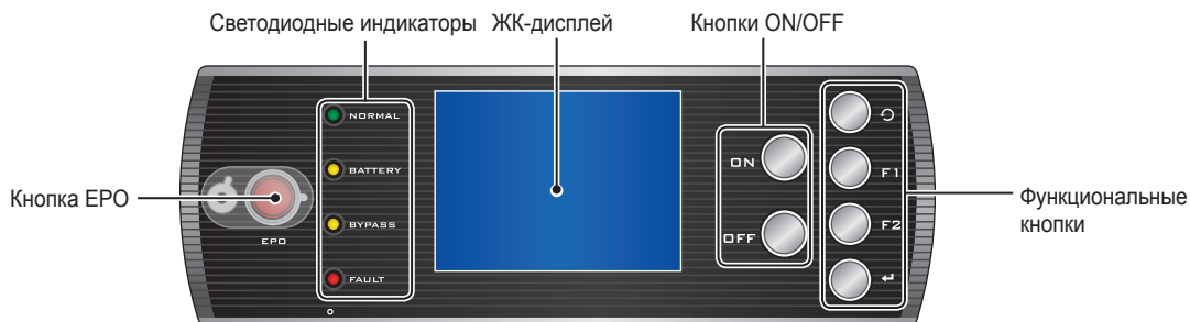
Рис. 2-8. Панель управления
