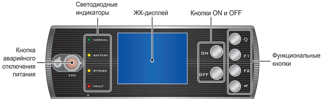
Рис. 7-2. Панель управления
