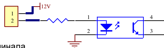
Рис.3-11 Схема REPO
