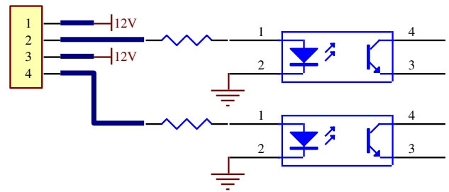
Рис.3-12 Входные контакты
