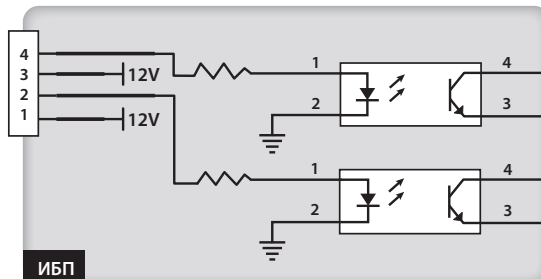
Рис. 4-6. Входы с сухими контактами (два комплекта)
