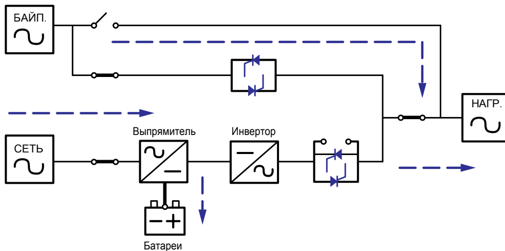
Рис. 4-5. Передача электроэнергии через ИБП в режиме байпаса
