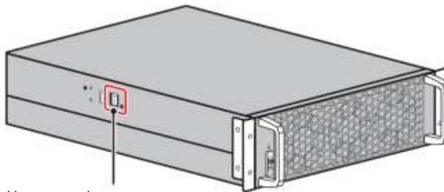
Рисунок 5-46: Нажатие на фиксатор силового модуля
