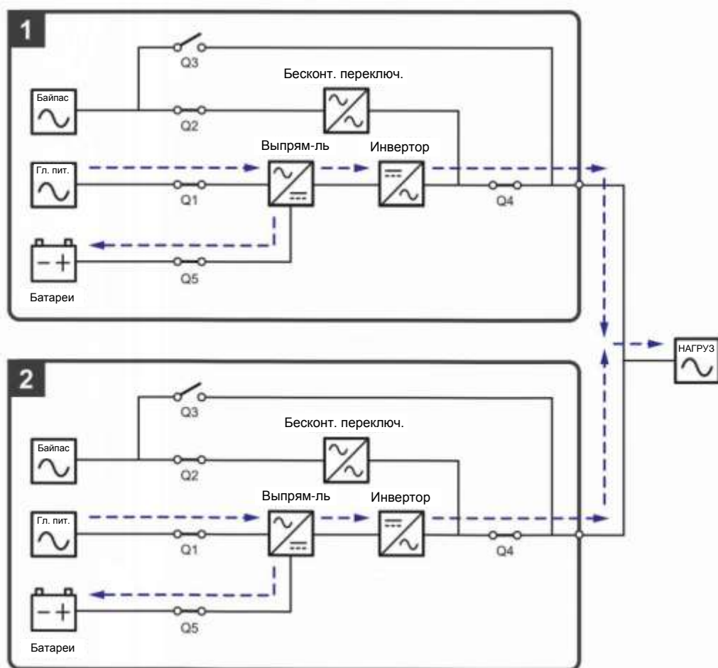
Рисунок 3-22: Схема режима двойного преобразования, подключение параллельных ИБП к двум линиям питания
