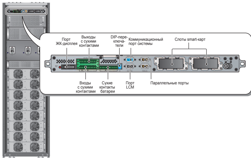
Рис. 2-12. Коммуникационные интерфейсы
