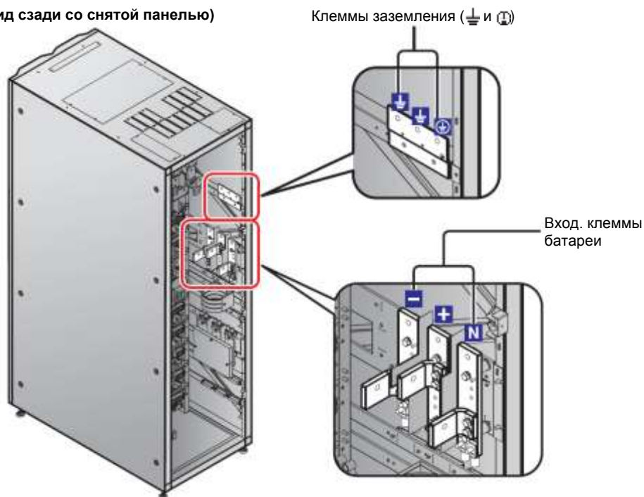
Рисунок 2-10: Клеммы: вход для подключения батарей и заземления
