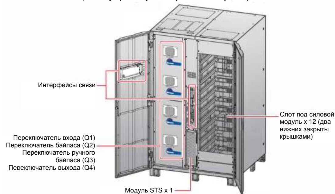
Рисунок 2-4: Вид ИБП внутри с открытыми дверцами
