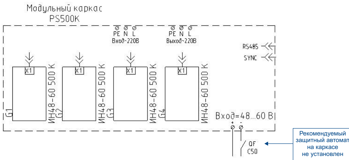
Инверторы Штиль PS48-60/500K в модульном каркасе PS500K
