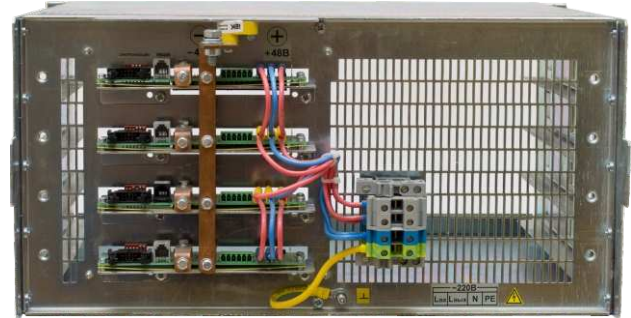
Модульный каркас Штиль PSI 4/1500 Вид с тыльной стороны
