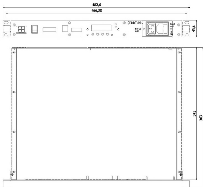
Инвертор PS60/1500, PS60/1500(STS)
