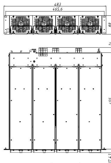
Модульный каркас PS2000K
