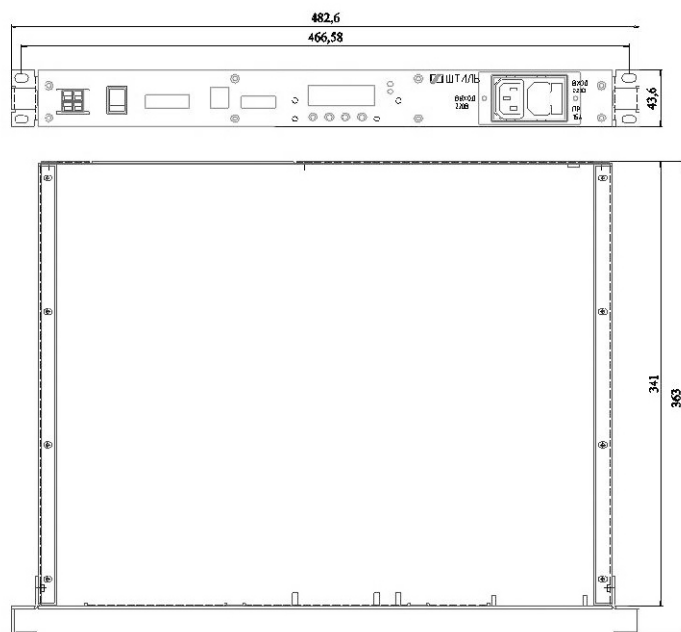
Инвертор PS48/1500, PS48/1500(STS)
