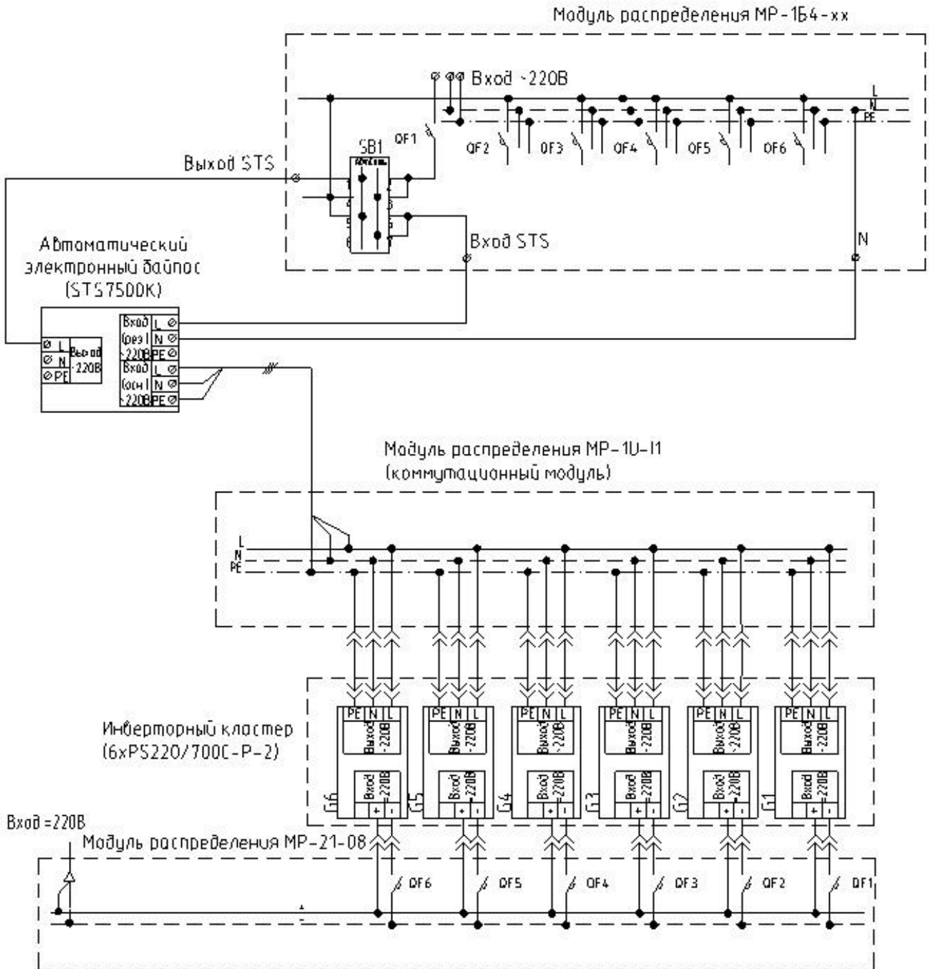
Инверторы Штиль серии С-Р с электронным байпасом, коммутационным модулем и модулями распределения
