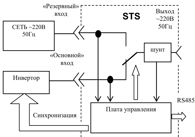
ON-LINE («основной» источник - Инвертор)
