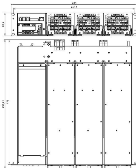
Модульный каркас PS2000KM
