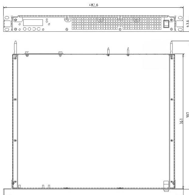
Инвертор PS60/1500(HS), PS60/1500(STS-HS)
