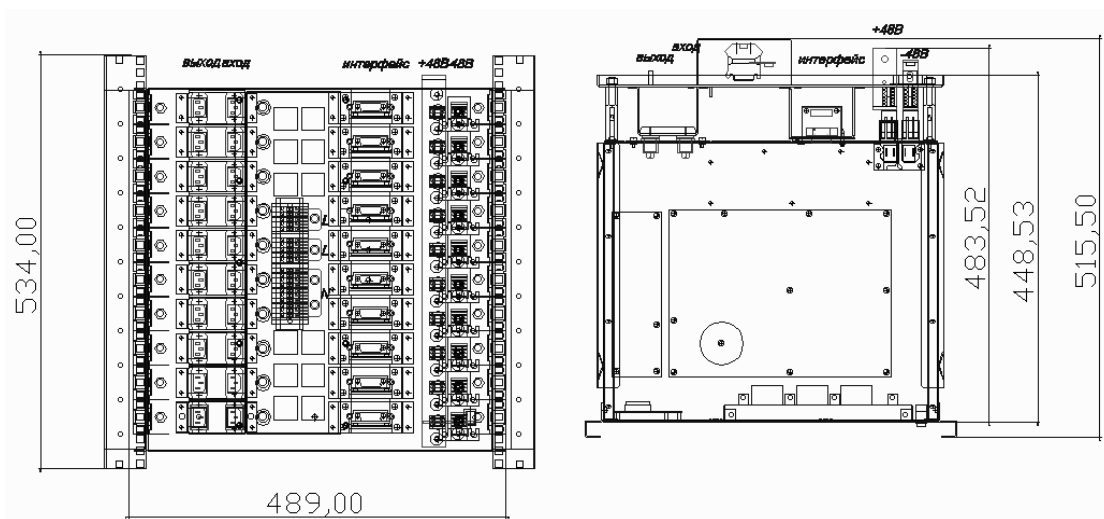
Модульный каркас Штиль PSI10/1500
