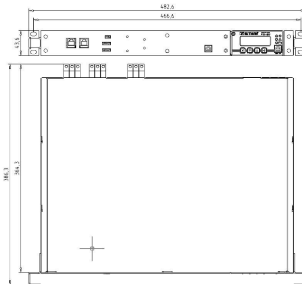
Электронный байпас Штиль STS3000K, STS7500K
