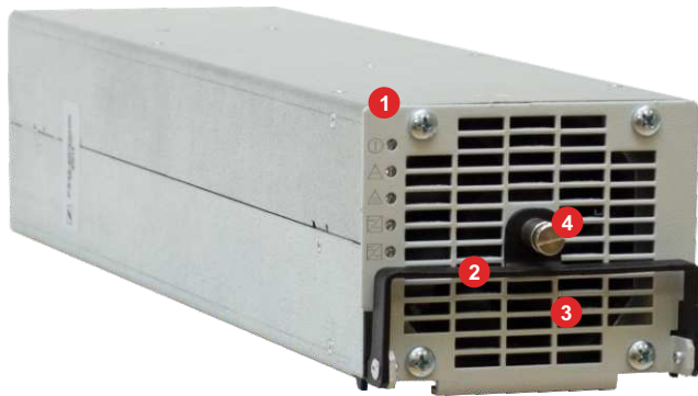
Инвертор Штиль PS220/2000K
