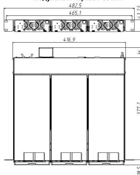
Модульный каркас PS1000K
