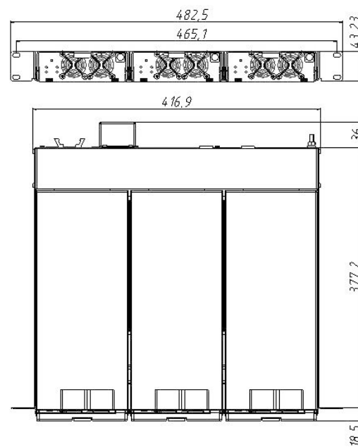
Модульный каркас PS1000K с 3-мя инверторами PS48-60/1000K
