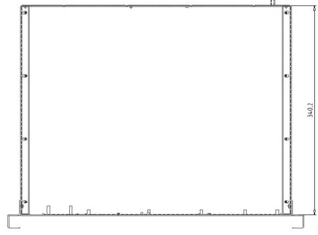
Инвертор PS24/700C-P-2
