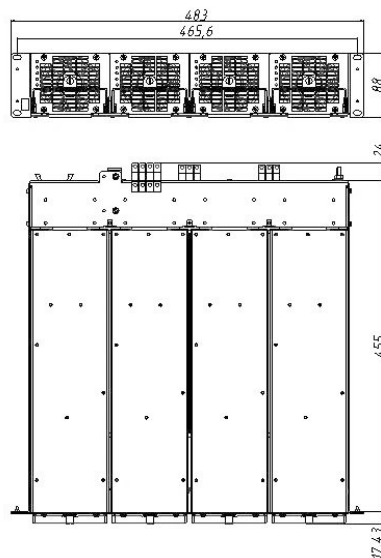
Модульный каркас PS2000K с 4-мя инверторами PS220/2000K
