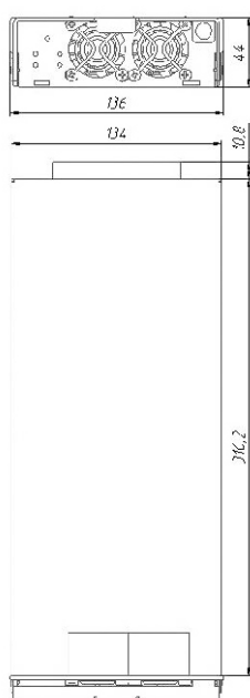
Инвертор PS48-60/1000K, PS48-60/1000K(I)
